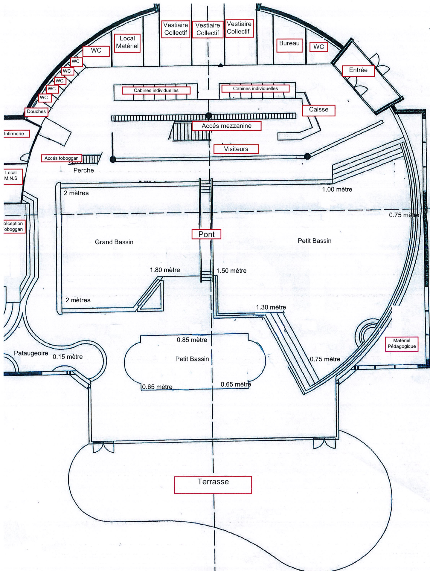
Plan RDC
